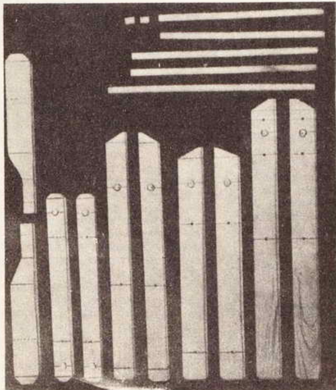
Tutte le parti occorrenti, prima di iniziare il montaggio della sedia. Una volta che tutte le parti maggiori saranno tagliate, in esse si praticheranno i fori occorrenti per i bulloni e per i rondini.
